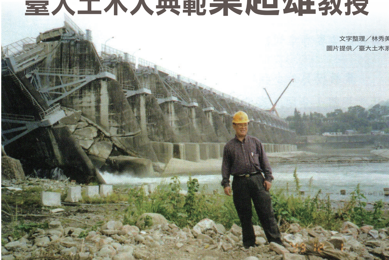
921大地震時進入災區勘災，於石岡壩。
