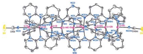
■ 圖 6b：2.3 奈米鉻九核金屬串錯合物的晶體結構。
