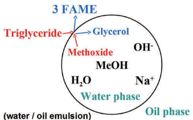
圖1：鹼催化三酸甘油酯甲基酯化反應的介面反應模式
