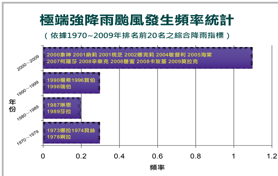
圖1：依據1970-2009年排名前20名之綜合降雨指標所定義之極端強降雨颱風發生頻率統計。
