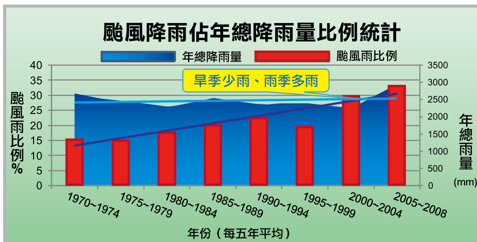
圖2：颱風降雨佔年總降雨量之比例統計，每五年平均。
