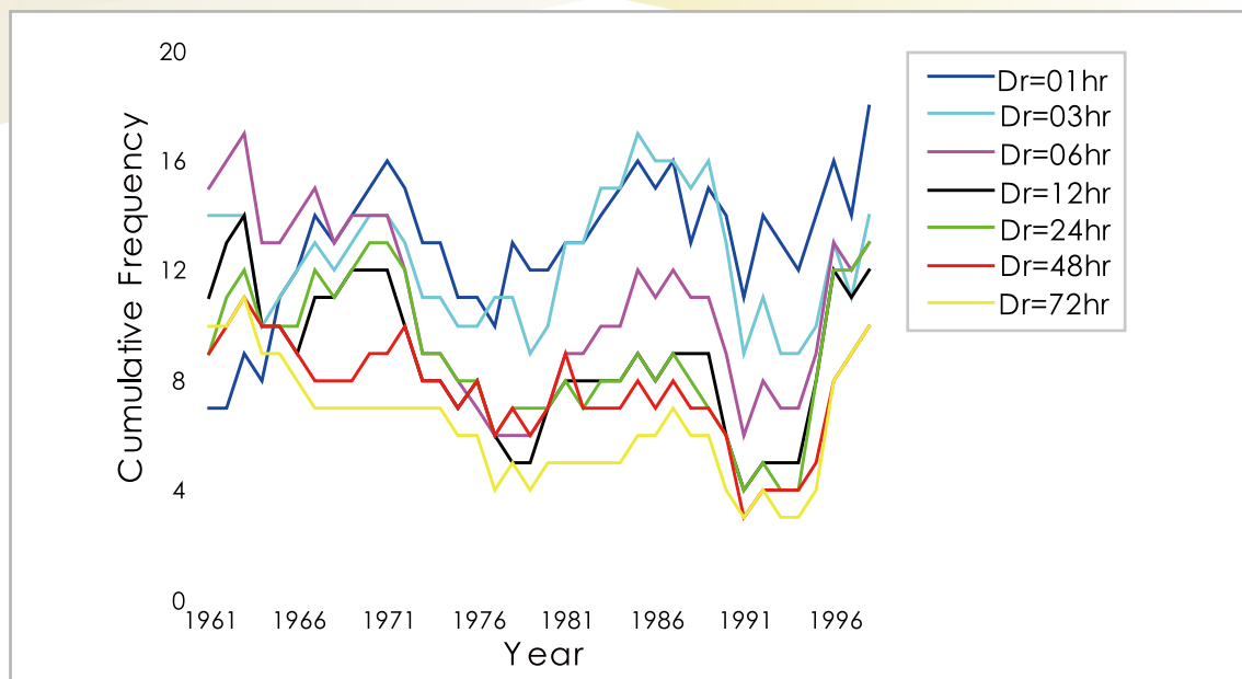
統計1961-1998年中部山區之阿里山、日月潭、玉山三個測站7種延時（1、3、6、12、24、48、72小時）重現期2年以上極端降雨事件的每10年的累積發生次數。雖然在1994年以後看到事件發生頻率明顯上升，但是在1994年以前的發生頻率也有高低變動，整體而言並沒有明顯的線性變化趨勢。
