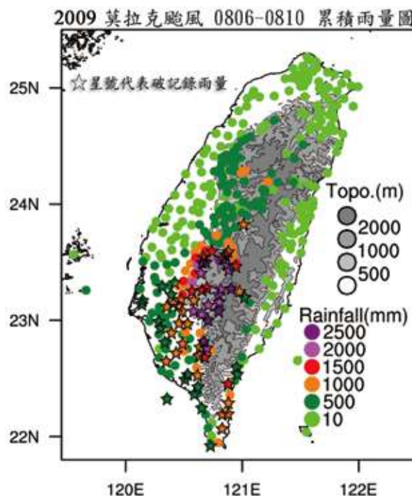
2009年8月6至10日莫拉克侵臺前後的5日累積雨量分布圖，極端（破記錄）降雨事件集中在臺灣南端山區與沿海區域，嘉義以北的西部沿海區域和臺東以北的東部沿海區域的5日累積雨量都在500毫米以下，突顯了極端氣候事件的地方特色。（製圖：氣象局 李明營）
