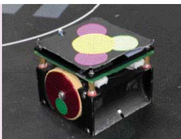
圖7 足球機器人外觀
