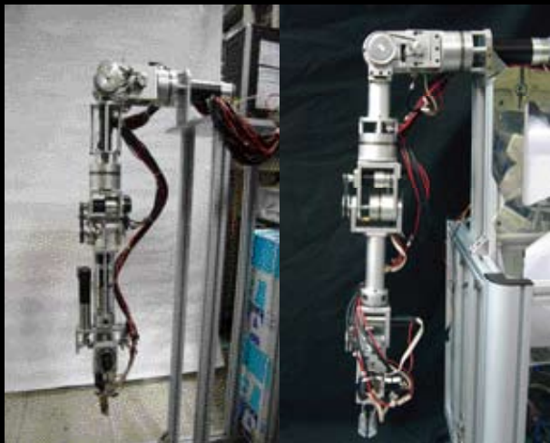
圖9 機構實體圖
