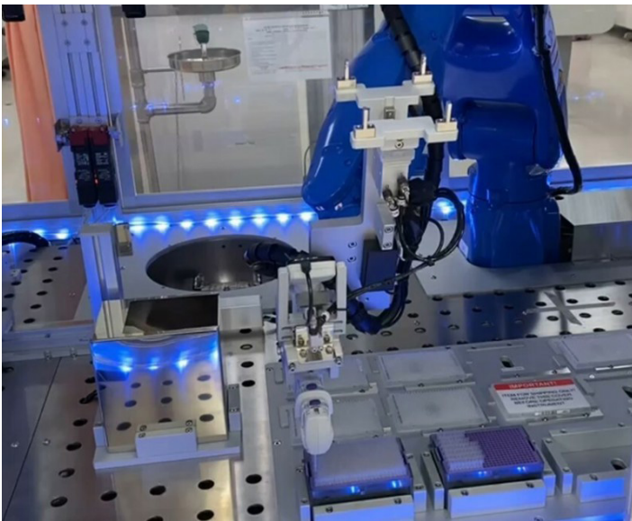
新竹臺大分院生醫醫院6月4日啟用「高通量全自動新型冠狀病毒核酸檢測系統」核酸萃取區之機械手臂執行自動分注試劑。（圖／新竹臺大分院提供）
