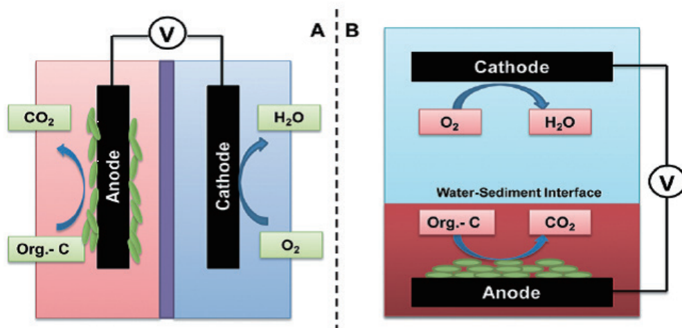
圖5：微生物燃料電池（A）與沉積物微生物燃料電池（B）比較（Xu et al., 2015）
