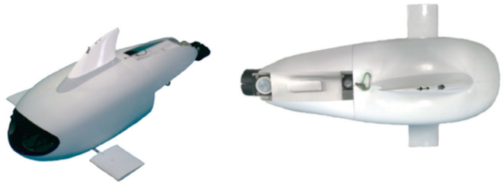
圖4：強力迴旋載具的側視（左）及俯視（右）圖。長90公分，重19.5公斤。使用艏旋螺槳與胸鰭剎車做高速迴轉，其迴旋半徑在航速每秒1公尺時為30公分。
